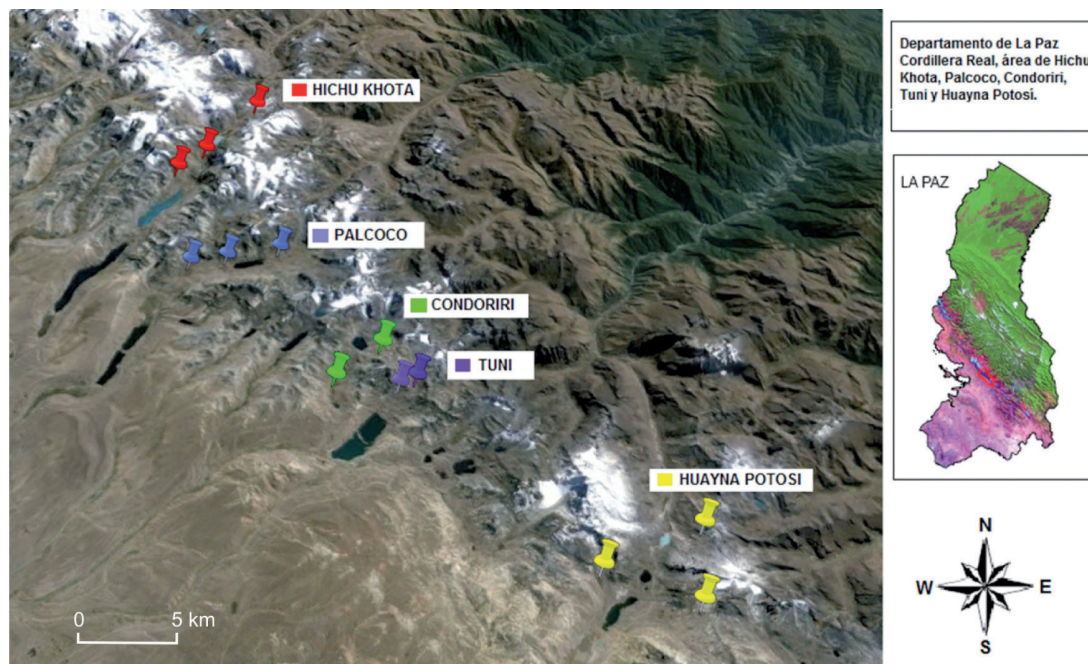
Figura 1. Mapa de ubicación del área de estudio (Izquierda: localización de la Cordillera Real en el Departamento de La Paz). Puntos de diferentes colores representan la pertenencia de cada uno de los bofedales estudiados en la cuenca glaciar (e.g., rojo: tres bofedales en la cuenca Hichu Khota).
